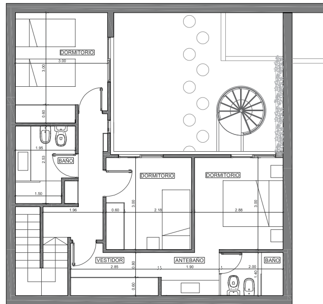
Planta Alta
