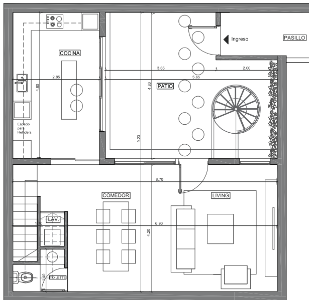
Planta Baja
