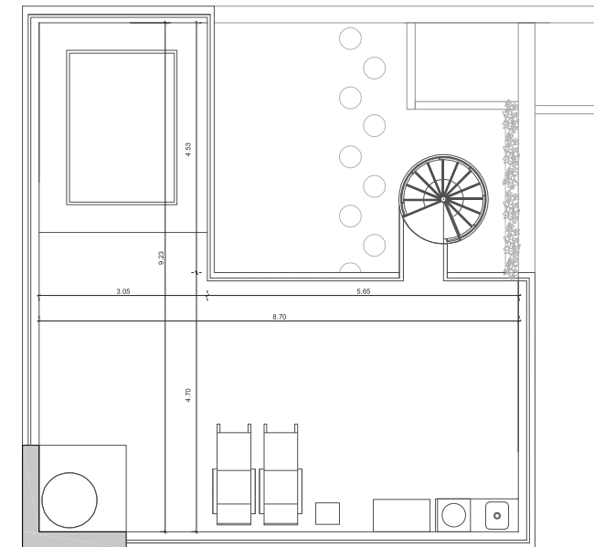
Planta Terraza
